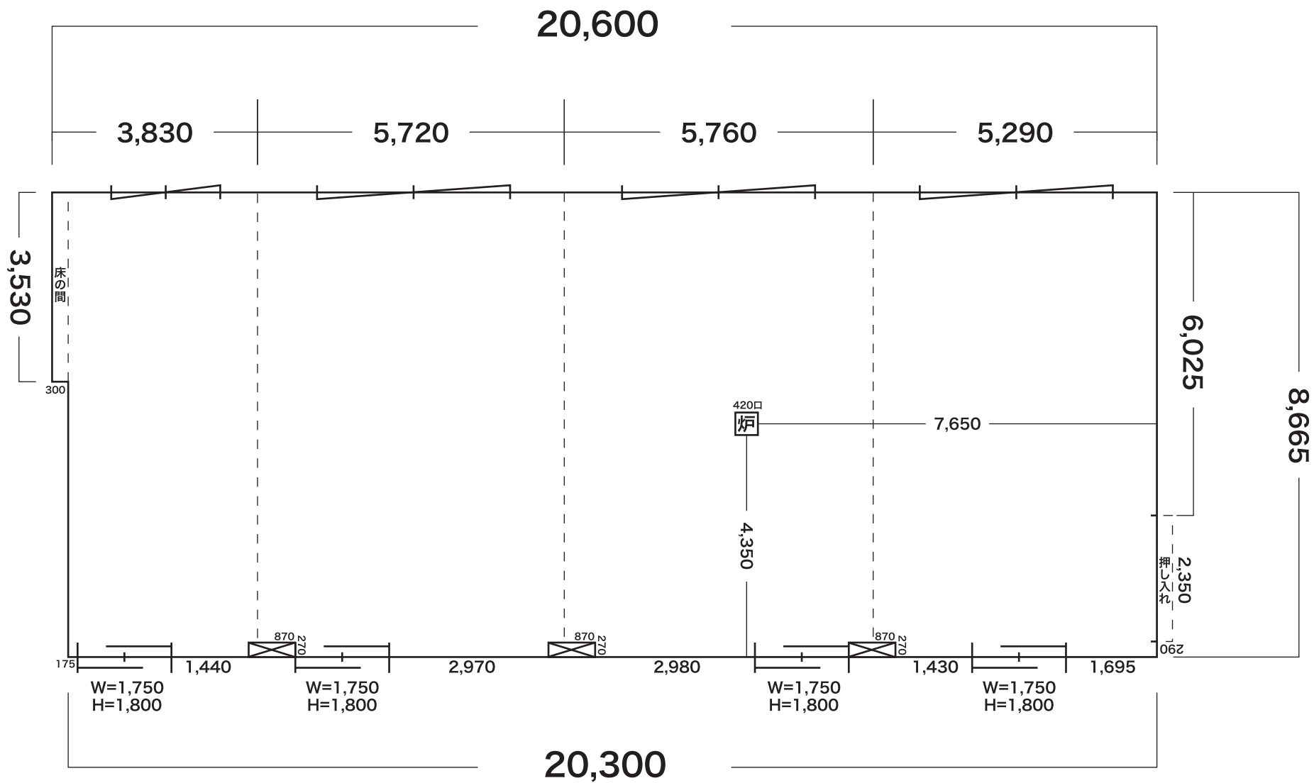
トーヨーホテル 4F 和室 1/100
