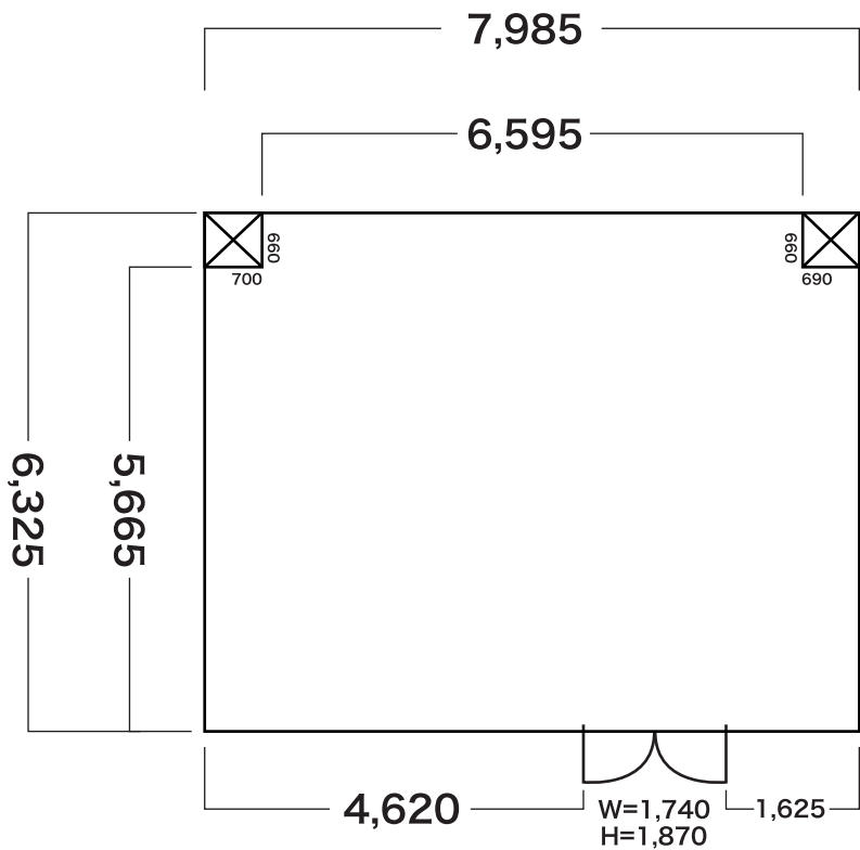
トーヨーホテル 3F サファイア 1/100
