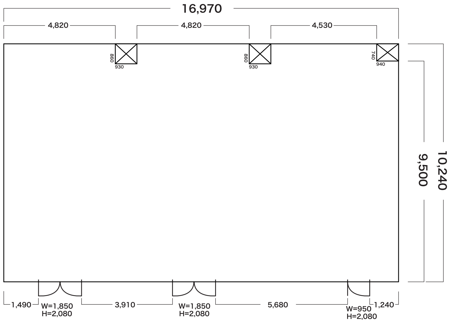
トーヨーホテル 3F 水晶の間 1/100 天井高 中央部 H=2,700 外周部 H=2,480
